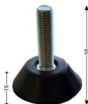
Lot de 4 pieds silentblocs
